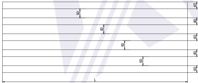
Hình 3: Mặt bằng thi công nhiều module trần U40
