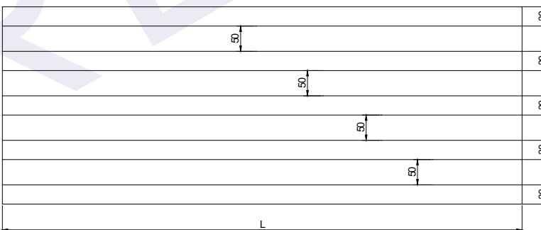
Hình 2: Mặt bằng thi công nhiều module trần U30 sử dụng xương trần U bước 80
