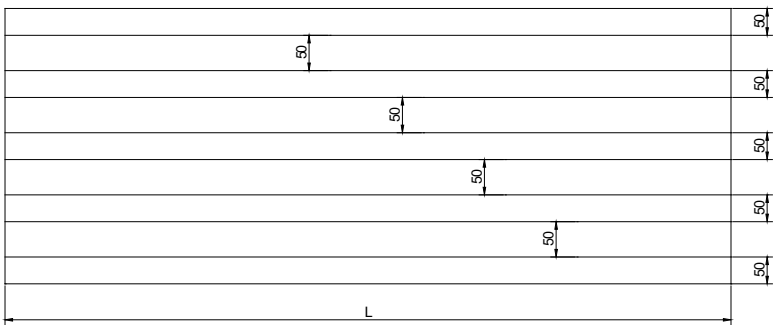
Hình 4: Mặt bằng thi công nhiều module trần U50
