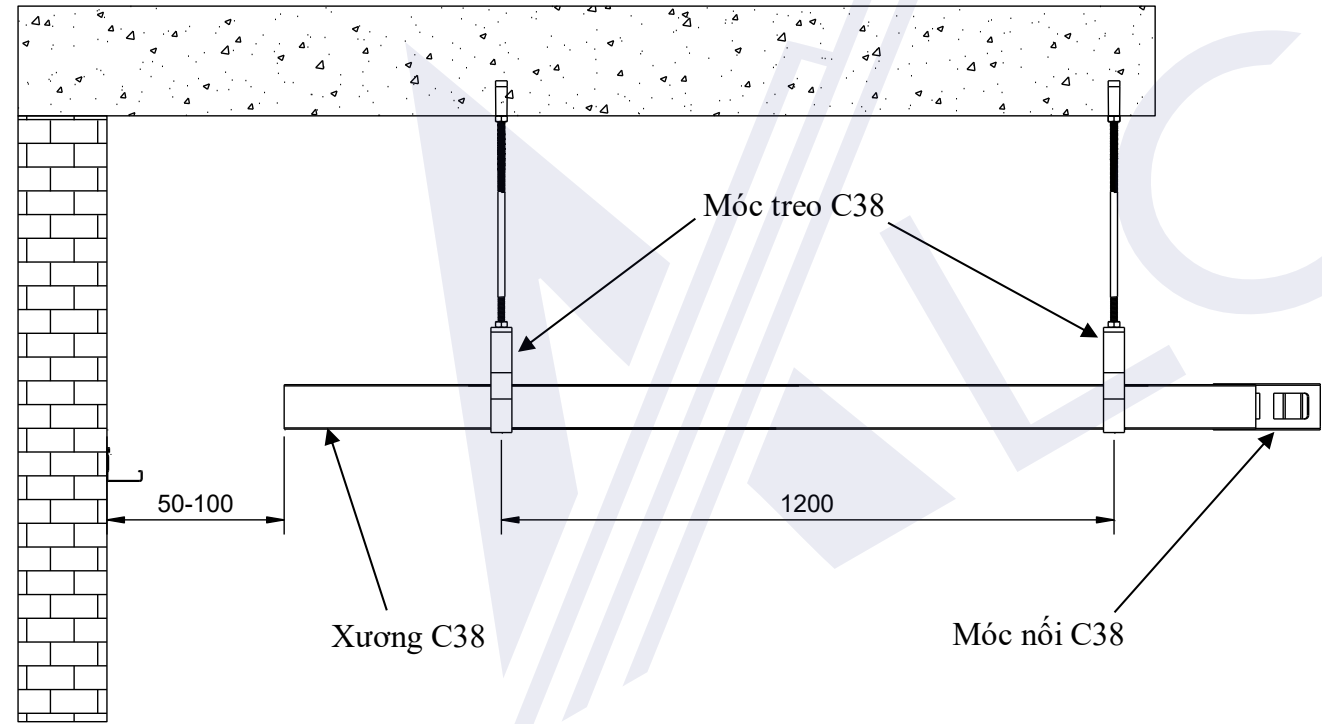
Hình 7: Lắp đặt khung xương C38
