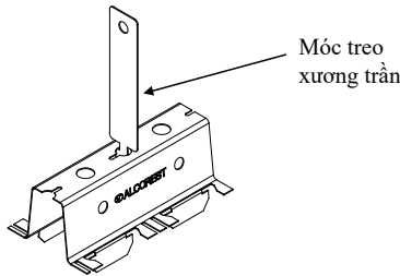
Bước 1: Lắp móc treo xương trần vào xương trần U
