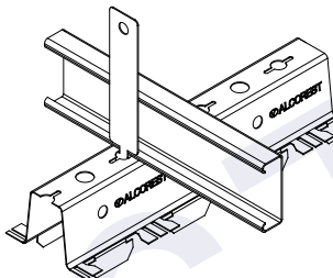
Bước 2: Áp lưng của xương trần U vào xương C38
