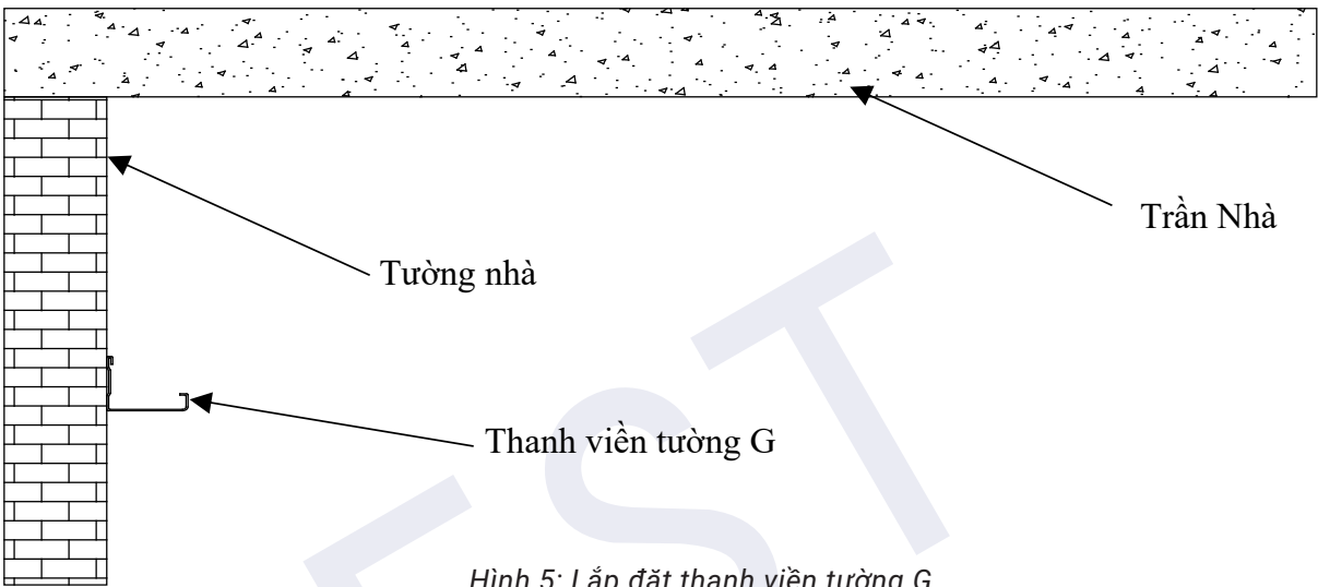
Hình 5: Lắp đặt thanh viền tường G
