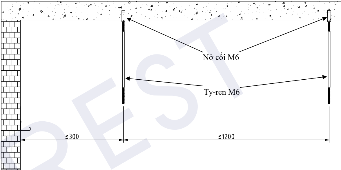
Hình 6: Treo thanh ty-ren lên trần
