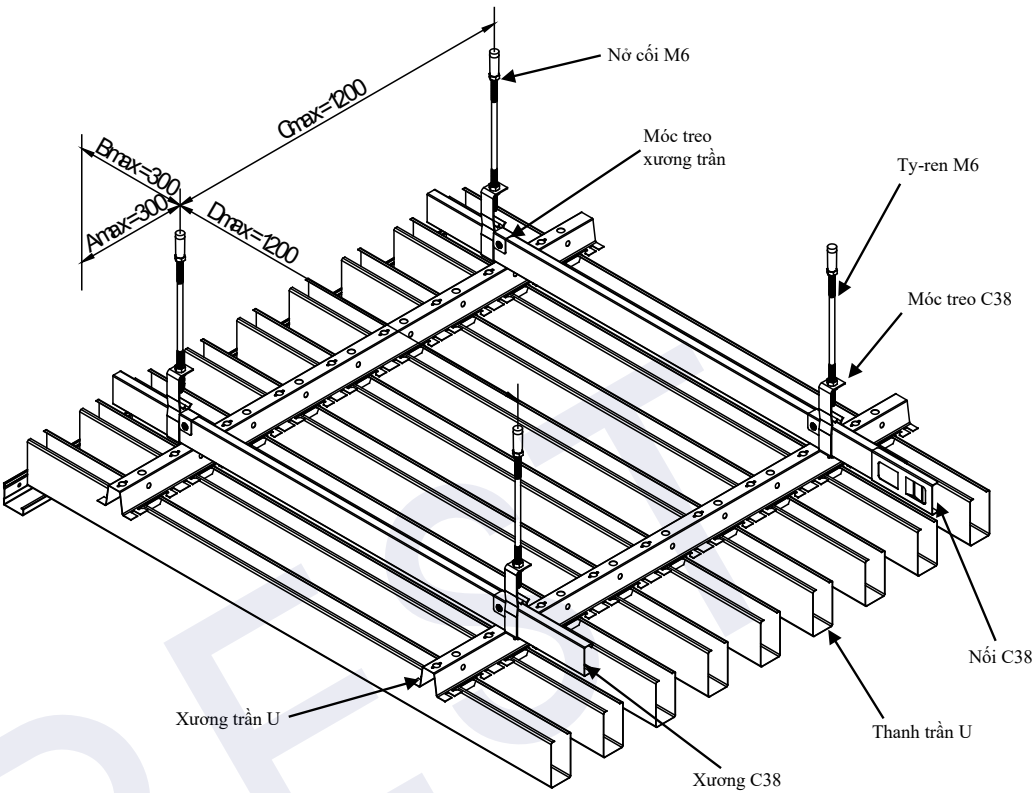
Hình 10: Hình ảnh lắp đặt hoàn thiện 1 module trần U
