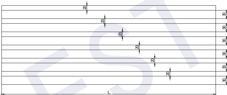
Hình 1: Mặt bằng thi công nhiều module trần U30 sử dụng xương trần U bước 50
