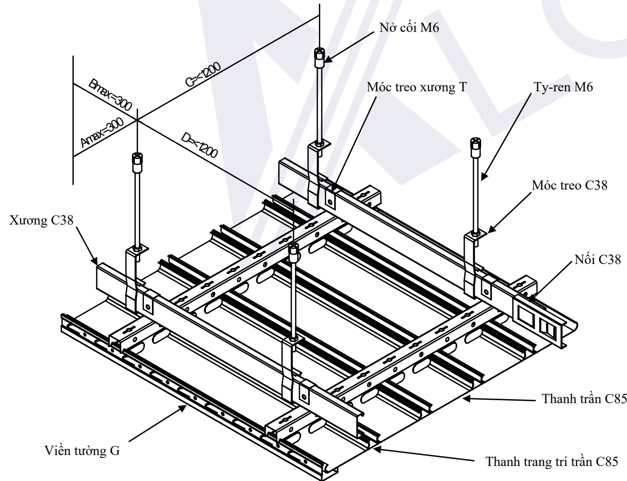
Hình 8: Lắp đặt hoàn thiện module trần C85
