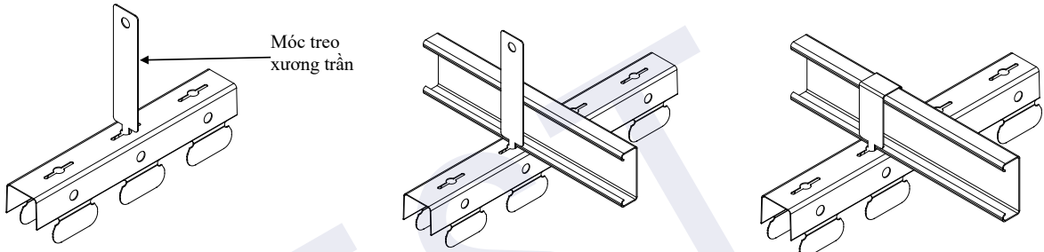
Bước 1: Lắp móc treo xương trần vào xương trần C85
