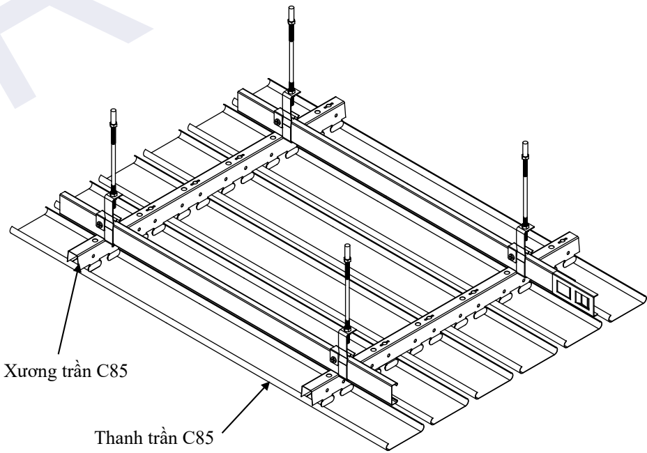
Hình 6: Lắp đặt thanh trần C85
